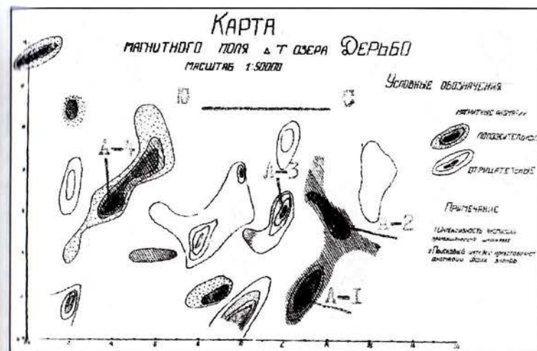
Мал. 3. Карта магнітнага поля возера Дзерба каля гарадзішча Маскавічы
