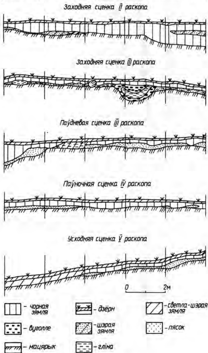
Рыс. 16. Профілі раскопаў на гарадзішчы Маскавічы
